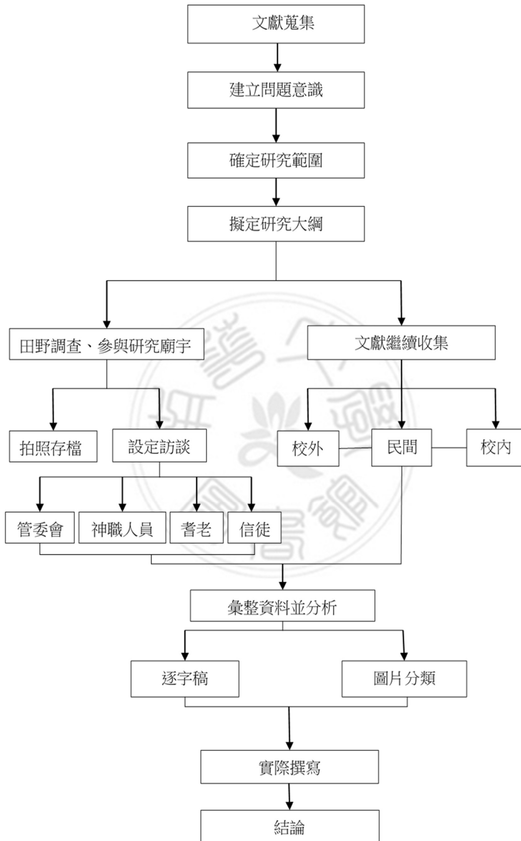
圖 3：研究流程圖
