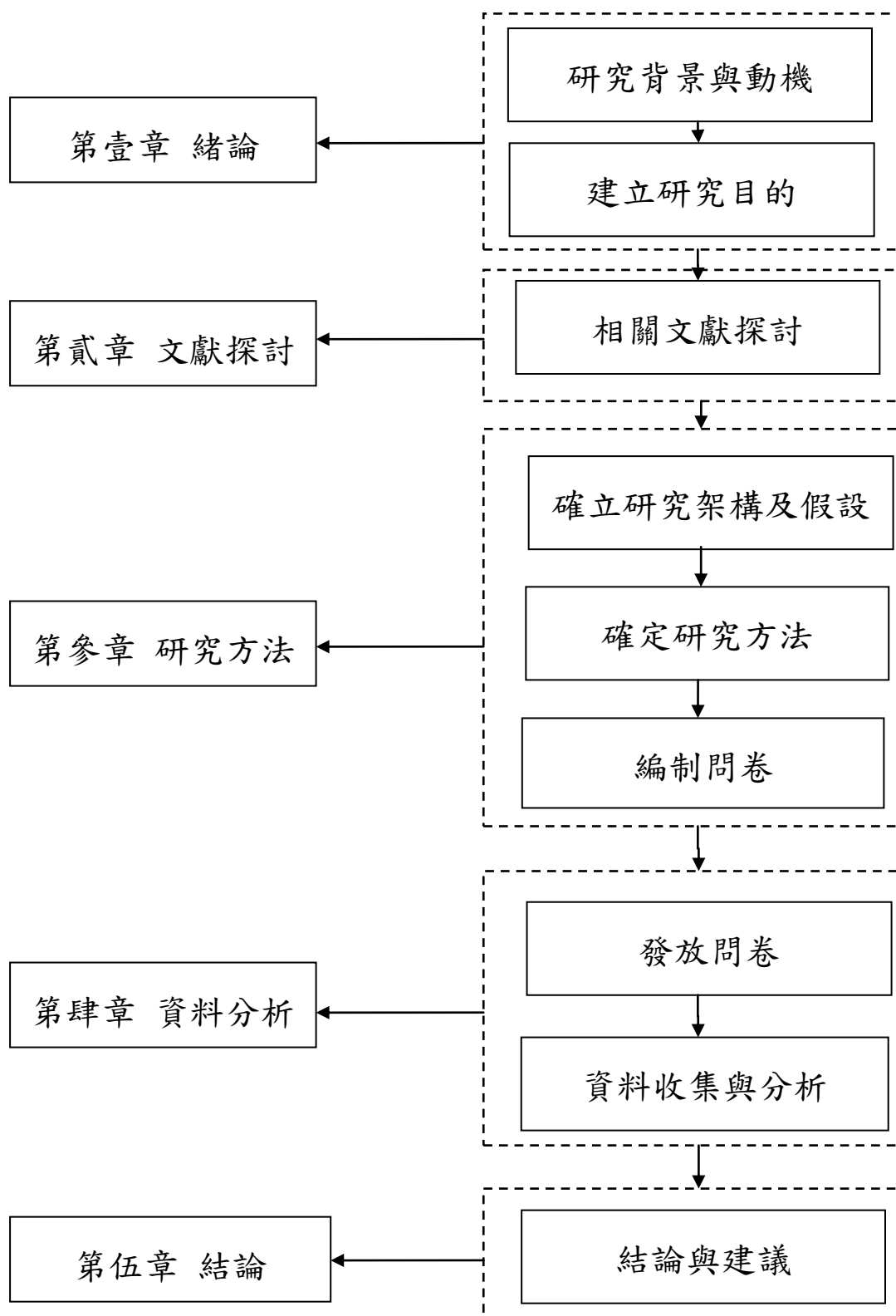
圖 1.5.1 研究流程
