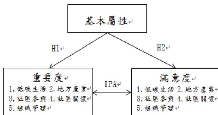
圖 3.1.1 研究架構圖
