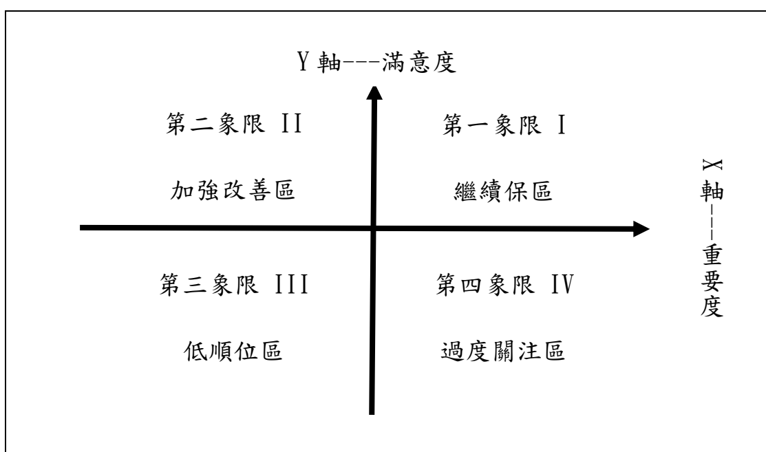
圖 4.6.1 IPA 象限圖
