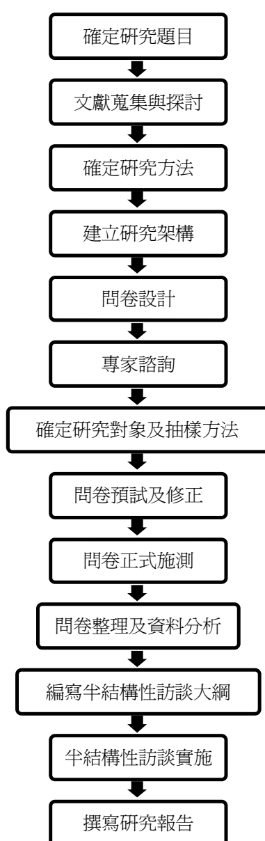
圖3-2 研究流程圖
