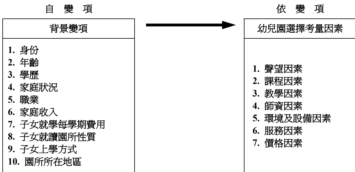
圖3-1、研究架構圖
