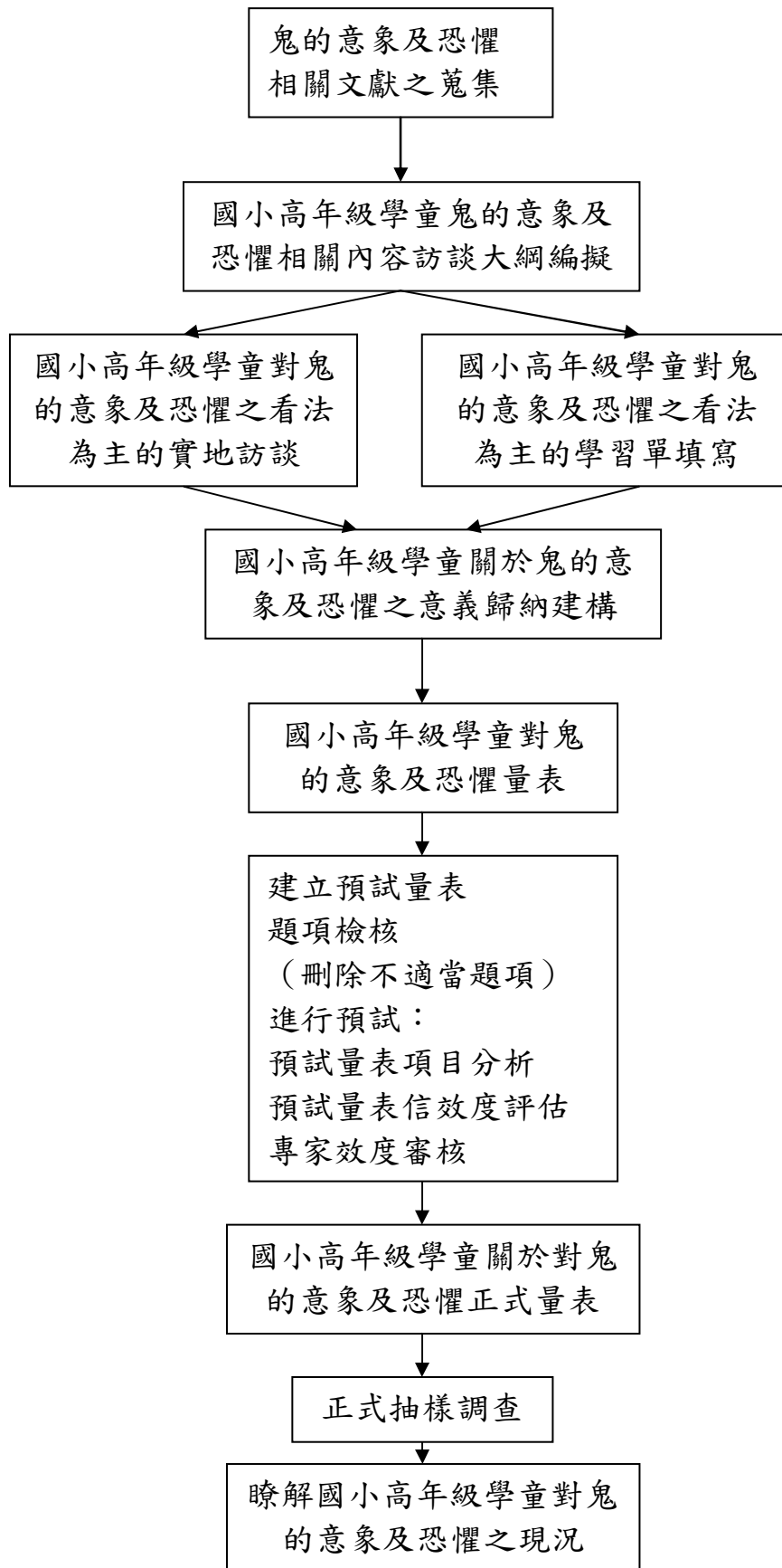
圖 3-3 研究流程
